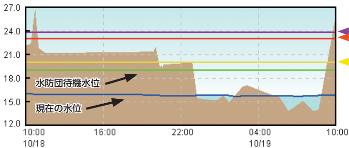
河川水位情報の例（信濃川） （所在地：長岡市信濃）
